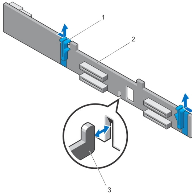
그림 35. 하드 드라이브 후면판 분리 및 설치
