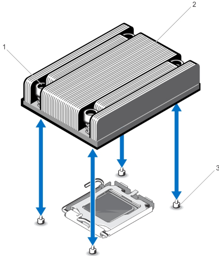
그림 29. 프로세서 방열판 분리 및 설치
