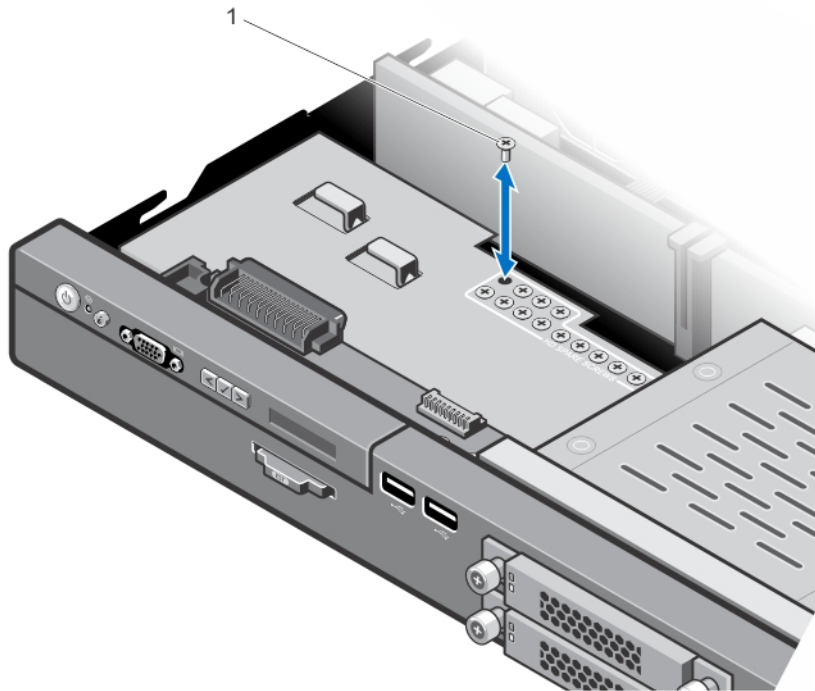
그림 18. 예비 하드 드라이브 나사 위치
