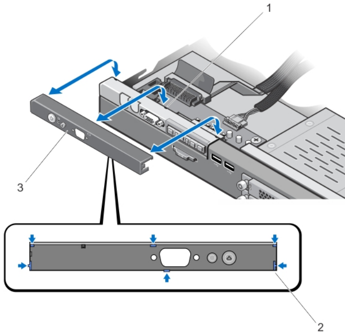
그림 37. 콘솔 분리 및 설치
