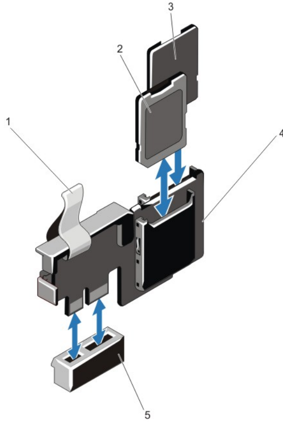
그림 27. 내부 이중 SD 모듈 분리 및 설치
