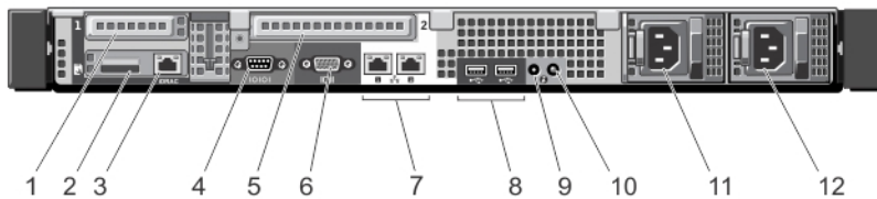
그림 4. 후면 패널 구조 및 표시등
