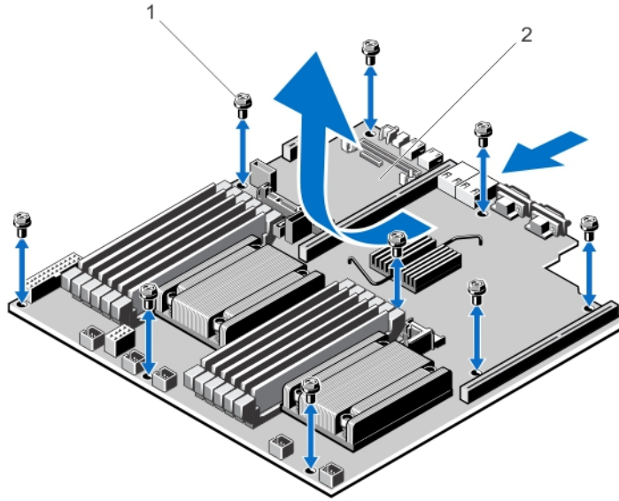
그림 41. 시스템 보드 분리 및 설치
