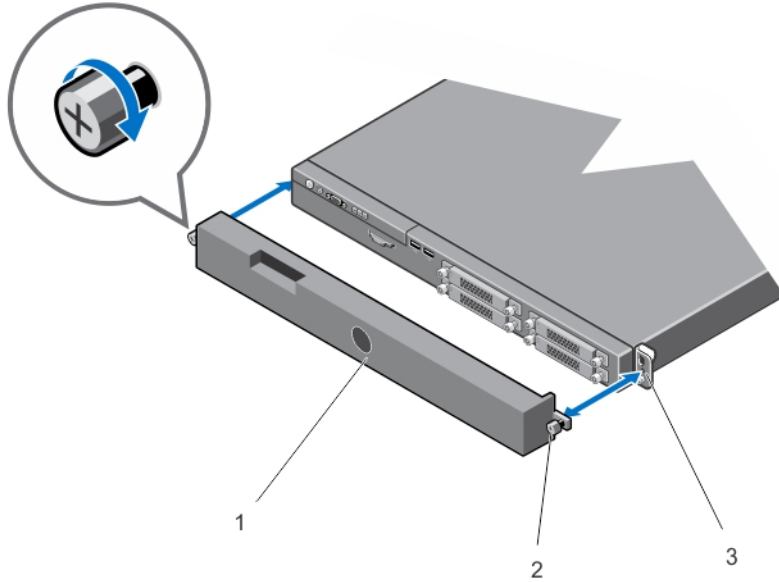
그림 7. 전면 베젤 설치 및 분리
