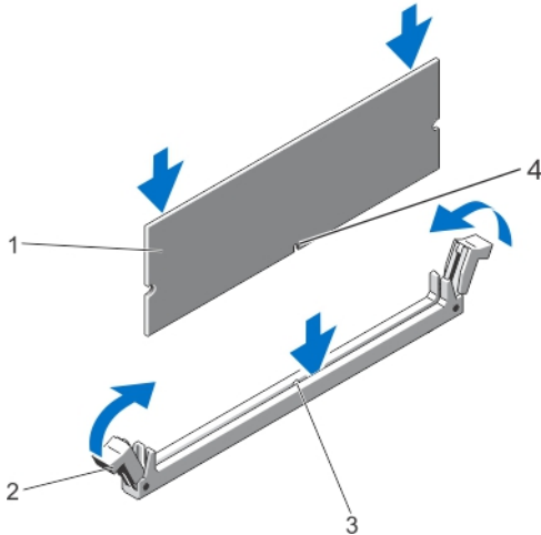
그림 15. 메모리 모듈 장착
