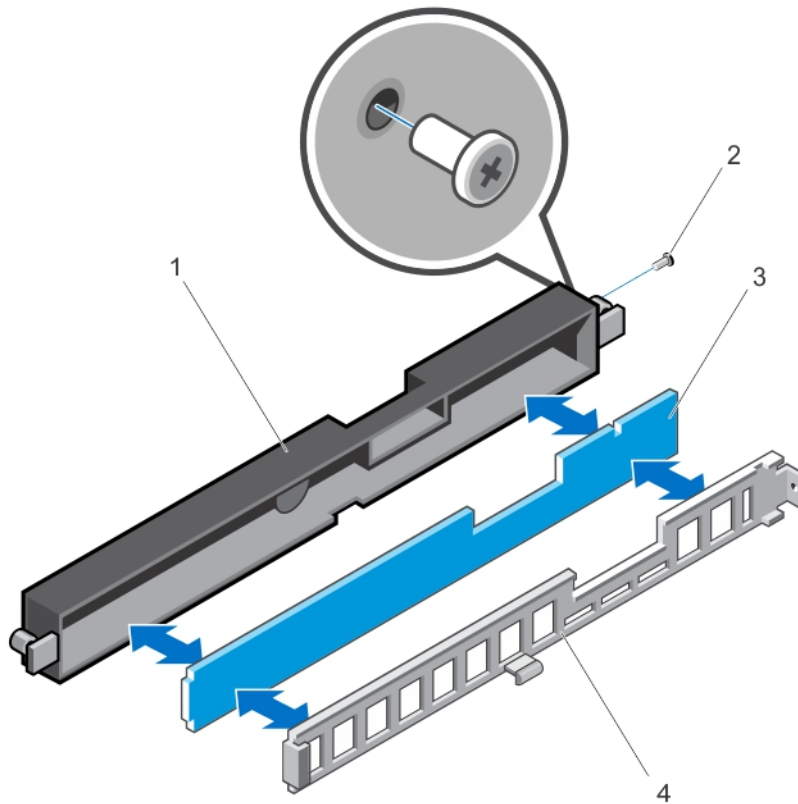
그림 8. 베젤 필터 분리 및 설치
