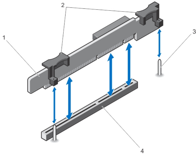
그림 23. 확장 카드 라이저 1 분리 및 설치
