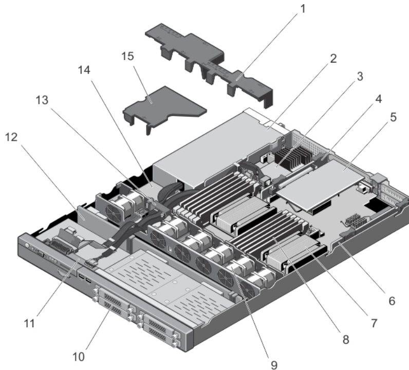
그림 10. 시스템 내부
