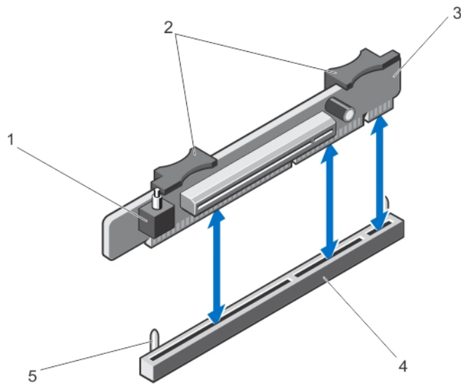
그림 24. 확장 카드 라이저 2 분리 및 설치
