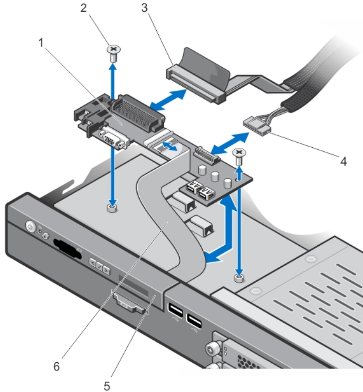
그림 38 . 제어판 모듈 분리 및 설치
