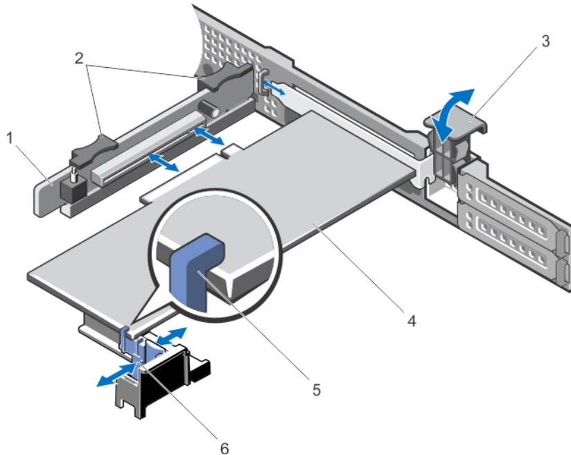
그림 22. 확장 카드 라이저 2에서의 확장 카드 분리 및 설치
