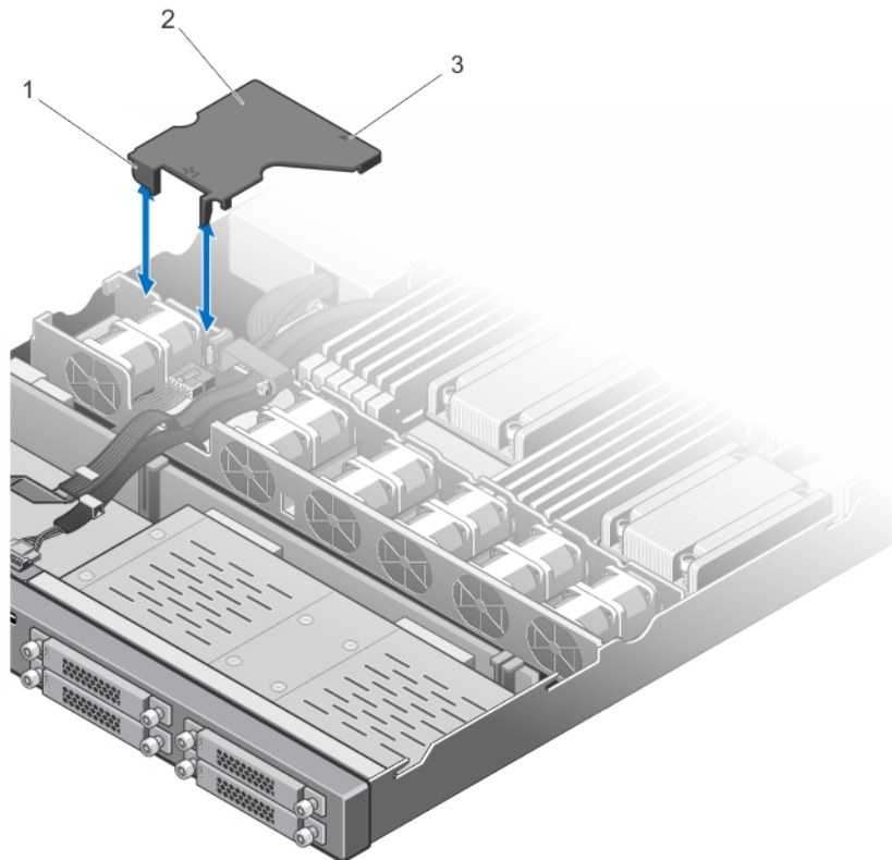
그림 39. PDB 덮개 분리 및 설치
