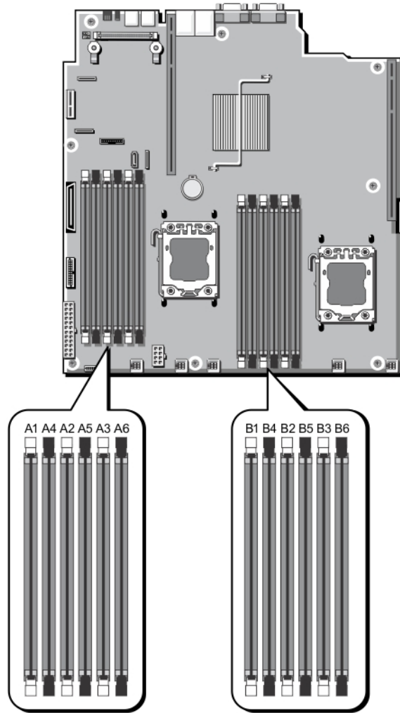
그림 12. 메모리 소켓 위치
