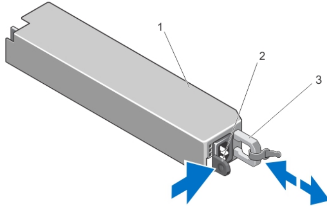
그림 31. 전원 공급 장치 분리 및 설치
