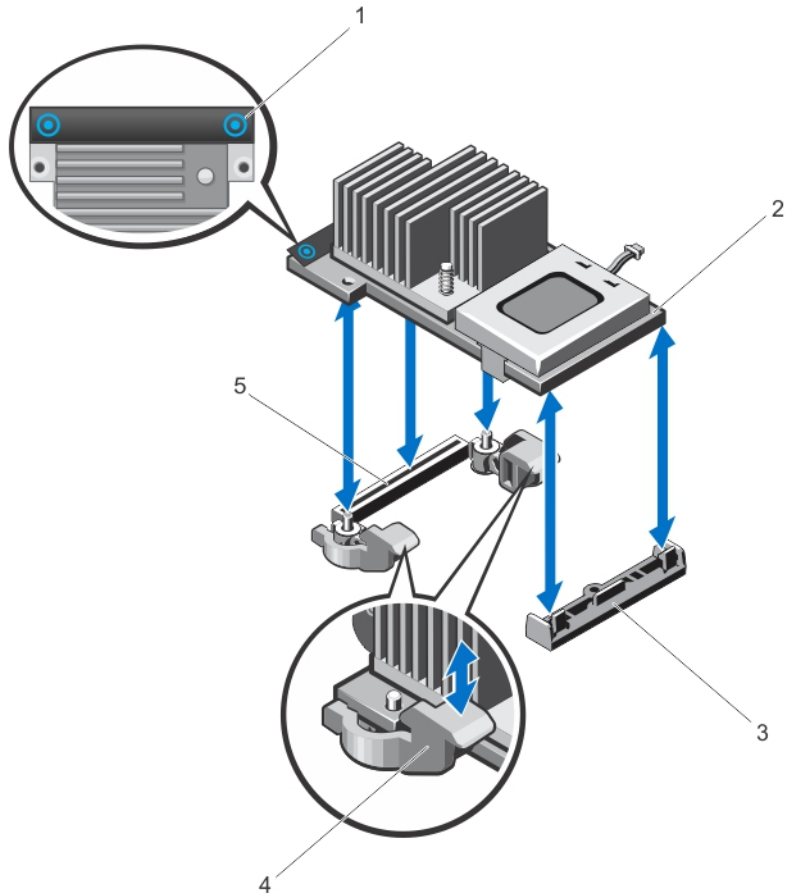
그림 28. 내장형 저장소 컨트롤러 카드 분리 및 설치
