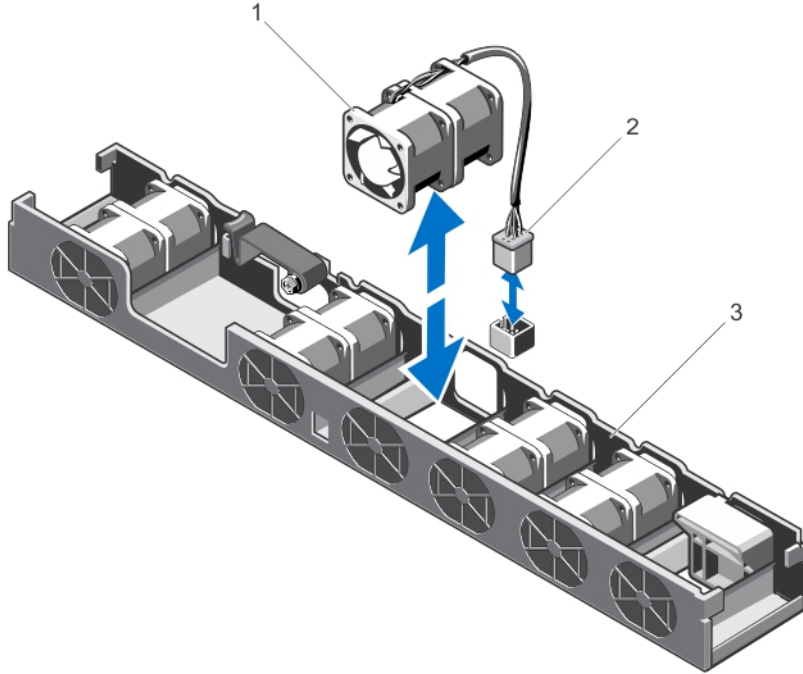
그림 19. 냉각 팬 분리 및 설치
