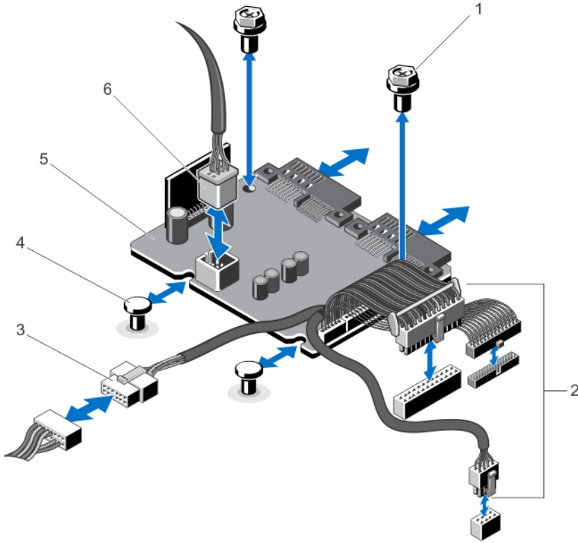
그림 40. 배전 보드 분리 및 설치
