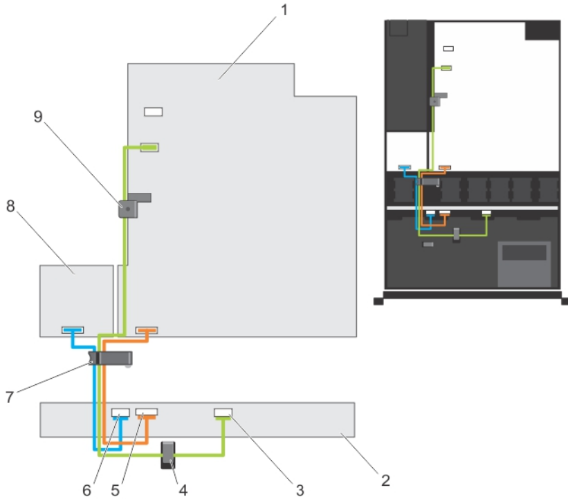
그림 36. 케이블 연결 다이어그램
