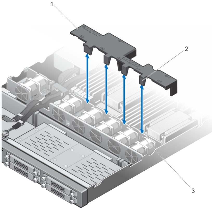
그림 11. 냉각 덮개 분리 및 설치
