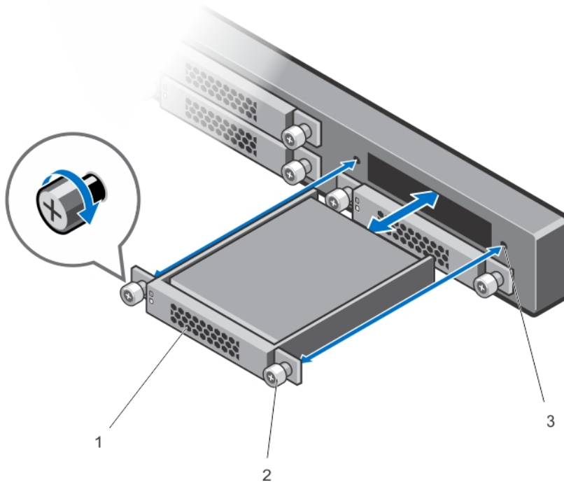
그림 16. 핫 스왑 하드 드라이브 분리 및 설치
