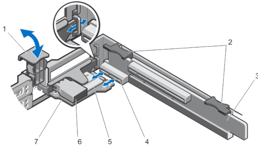
그림 25 . iDRAC Enterprise 카드 분리 및 설치
