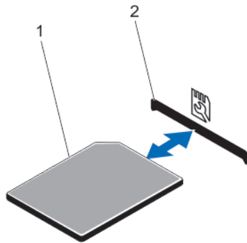
그림 26 . SD vFlash 카드 분리 및 설치
