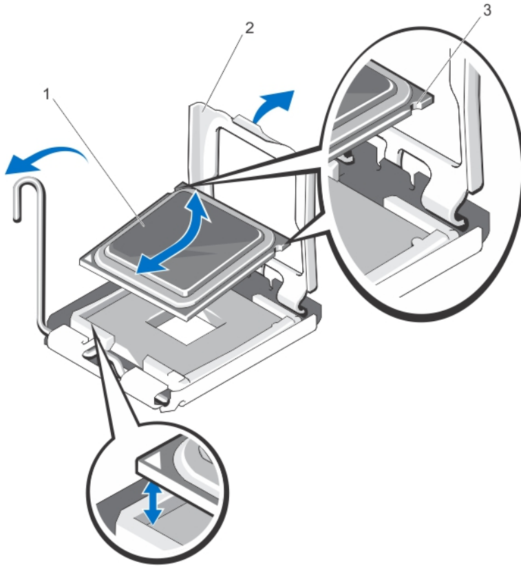
그림 30. 프로세서 분리 및 설치
