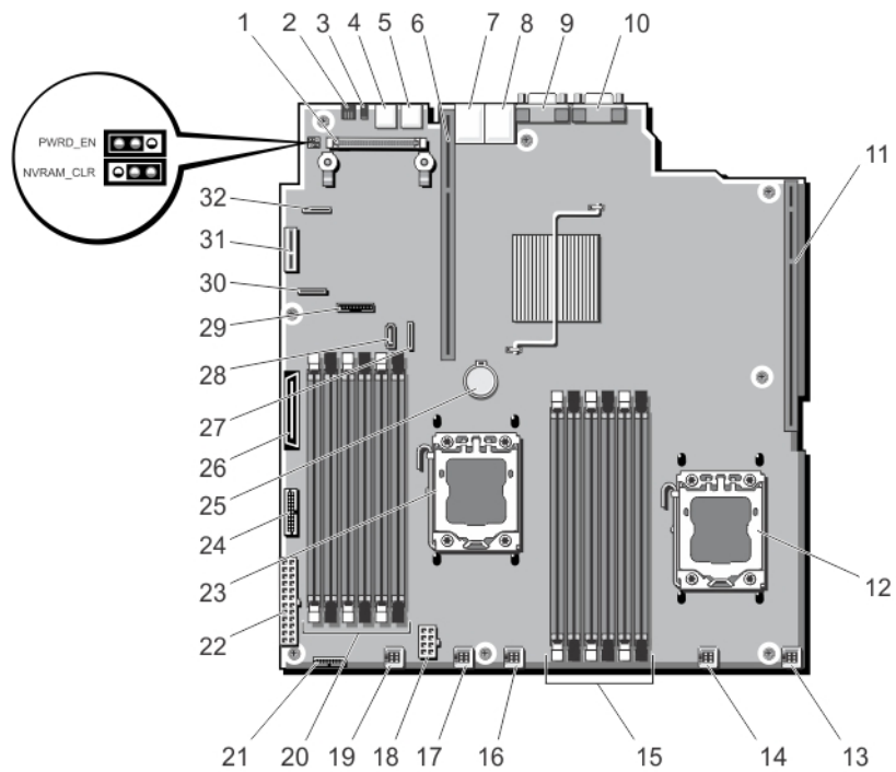
그림 42. 시스템 보드 접퍼 및 커넥터
