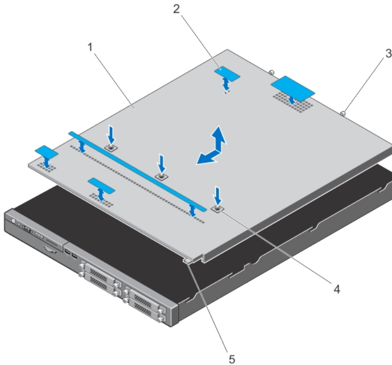
그림 9. 시스템 열기 및 닫기
