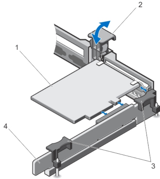
그림 21. 확장 카드 라이저 1에서의 확장 카드 분리 및 설치
